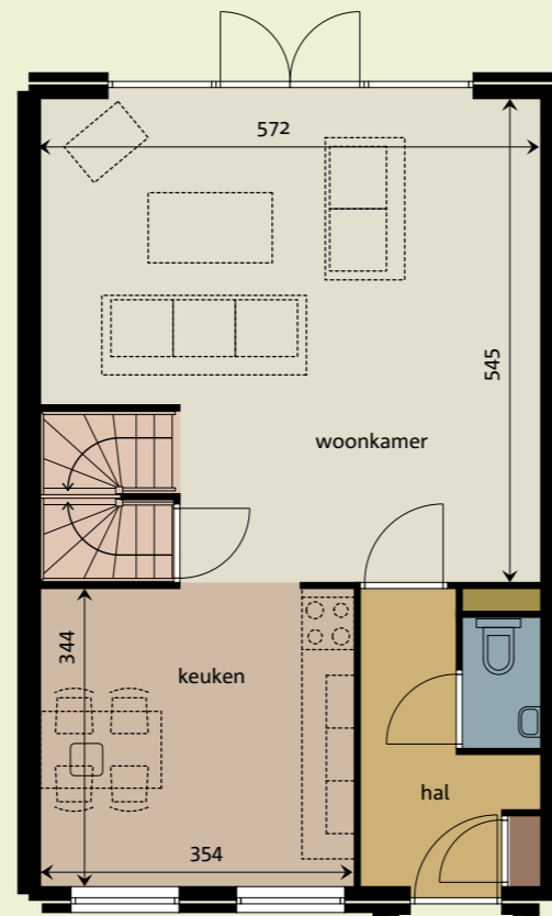
Begane grond
