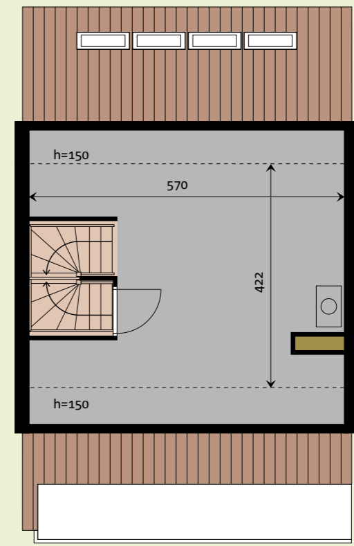
Tweede verdieping
