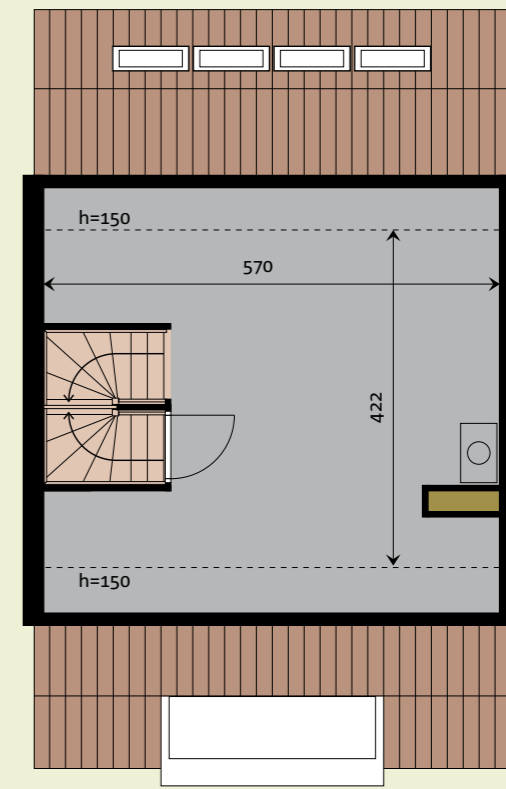
Tweede verdieping
