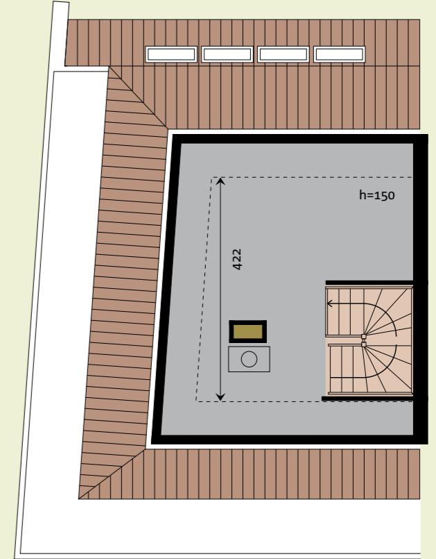
Tweede verdieping
