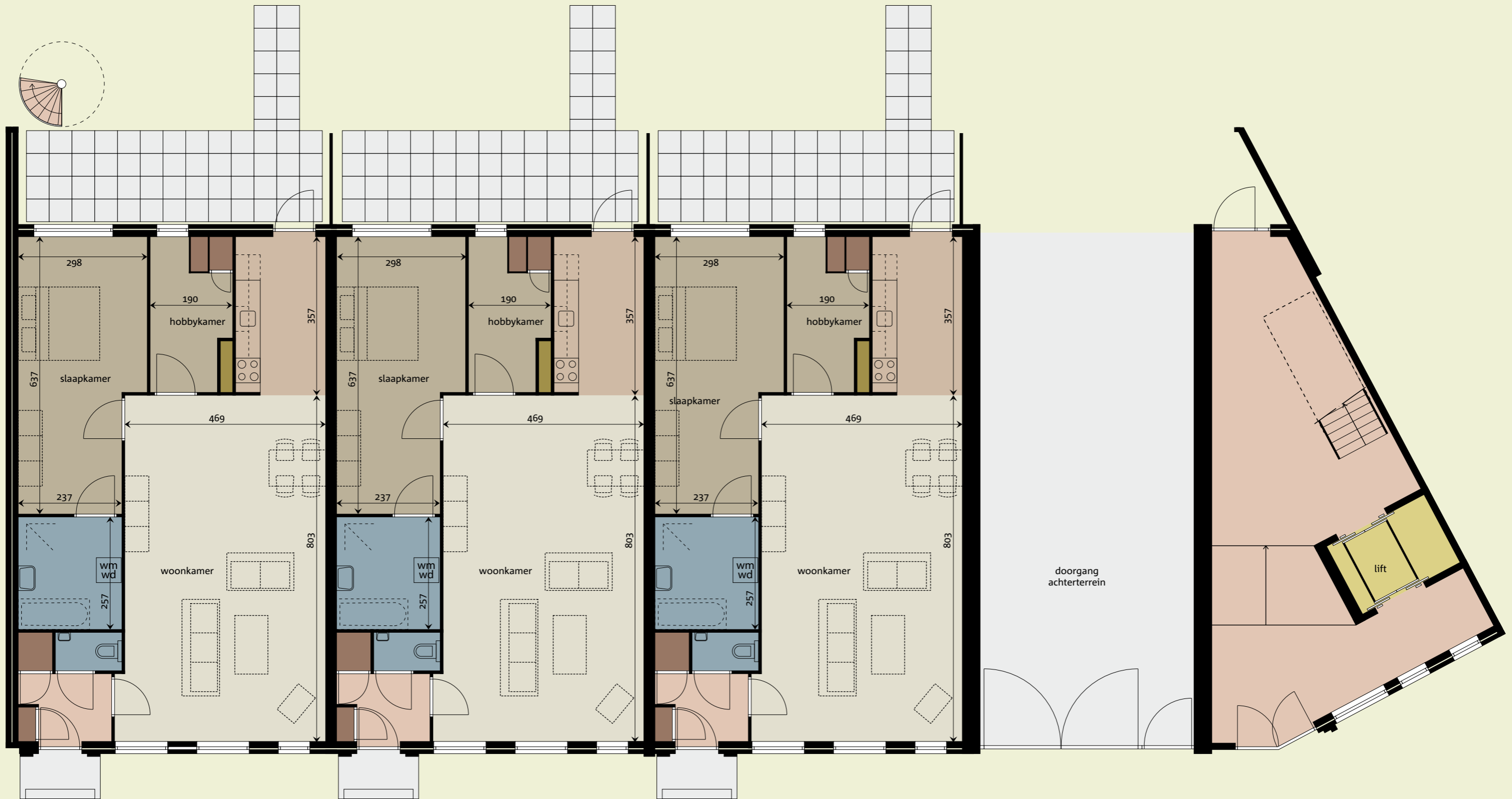
Appartement type S1
