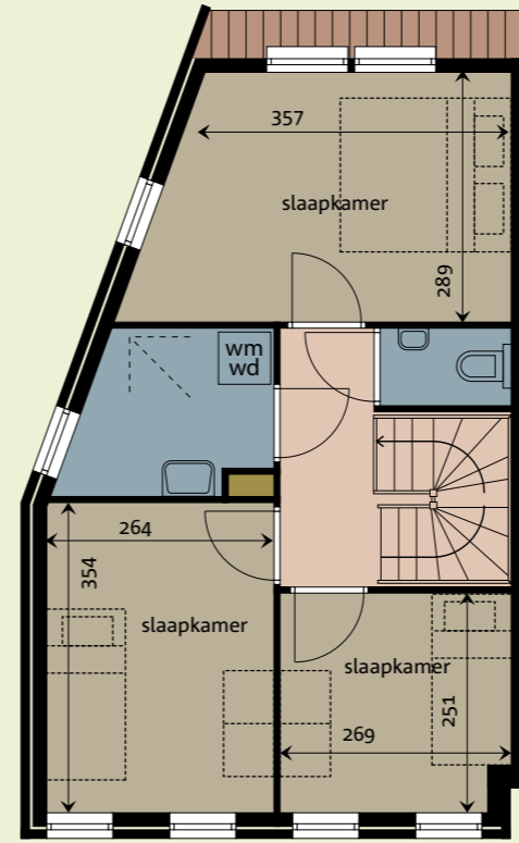
Eerste verdieping
