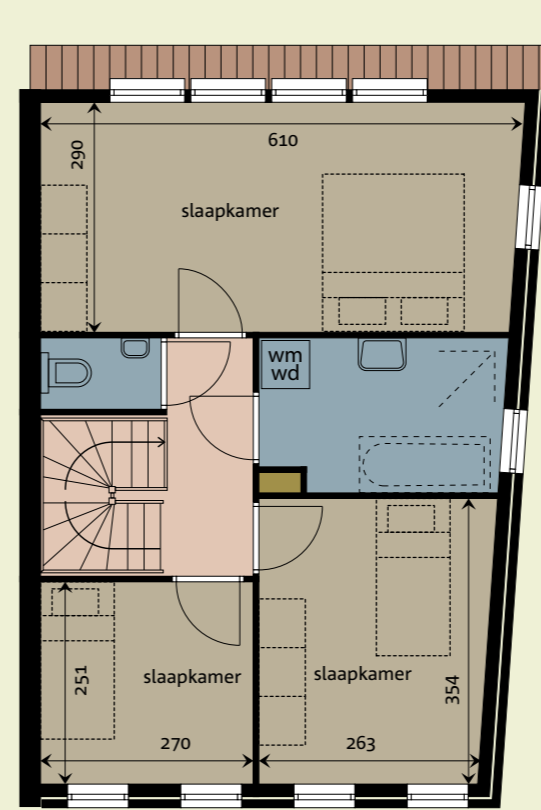
Eerste verdieping
