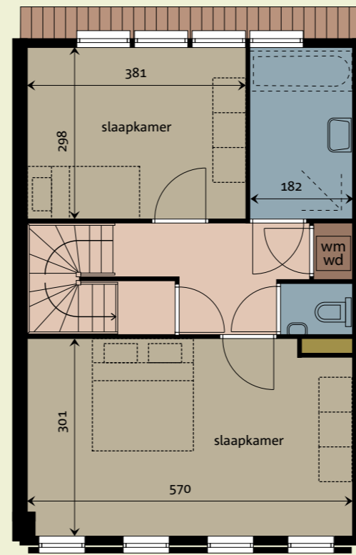
Eerste verdieping
