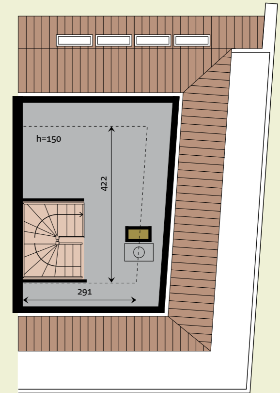
Tweede verdieping
